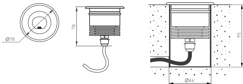
Рис. 1. Чертеж и габаритные размеры
