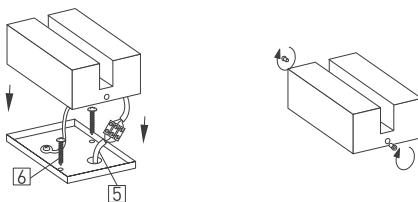
Рис. 4. Установка и подключение светильника на ровной поверхности
