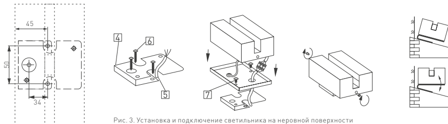
Рис. 3. Установка и подключение светильника на неровной поверхности
