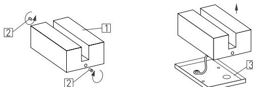
Рис. 2. Подготовка светильника к установке
