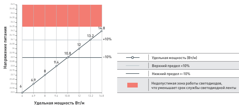
График 1. Зависимость удельной мощности от напряжения питания
